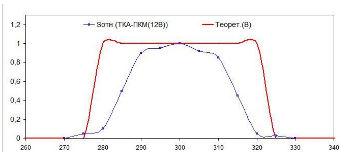
Рис.1 Относительная спектральная чувствительность прибора
