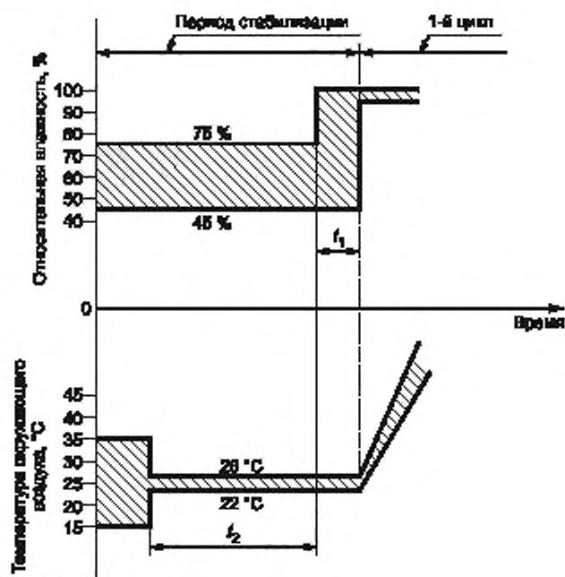
t_1 — время, требуемое для достижения 95–100 % относительной влажности (не превышающее 1 ч); t_2 — время, требуемое испытываемому образцу, чтобы достичь температурной стабильности
