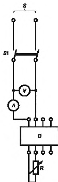
S — источник питания; SI — двухполюсный выключатель; V — вольтметр; A — амперметр; D — АВДТ; R — переменный резистор
