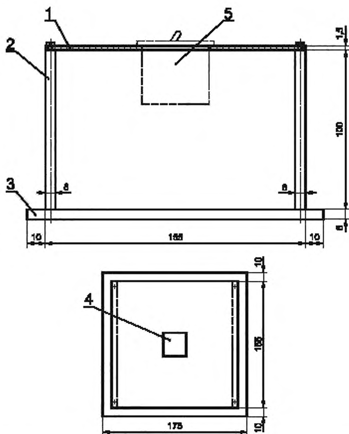
1 — съемная стальная пластина; 2 — алюминиевая пластина; 3 — монтажная плита; 4 — окно в стальной пластине для АВДТ; 5 — АВДТ
