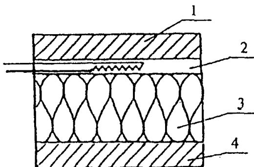
1 - нагреватель; 2 - тепломер; 3 - испытываемый образец; 4 - холодильник
