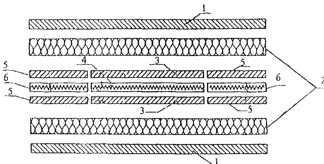
Рисунок А.2 - Схема прибора с двумя тепломерами
