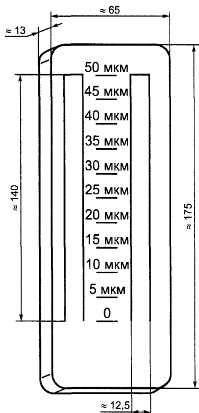
Рисунок 1 — Типовой прибор ( гриндометр )
