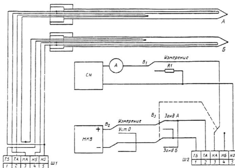
Рисунок 1 - устройство зонда и электрическая схема соединения приборов
