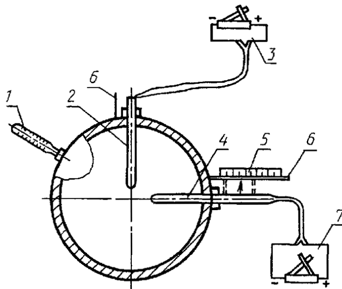
1 - термометр; 2, 4 - контрольная и рабочая напорные трубки, 3, 7 - микроманометры для измерений динамического давления в контрольной и рабочих точках; 5 - линейка; 6 - стальной пруток
