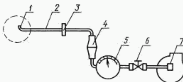
Заборное устройство
