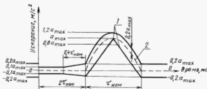
1 — пределы отклонений; 2 — номинальный пробег; a_{max} — пиковое ускорение удара; t_{ном} — длительность ударного импульса
