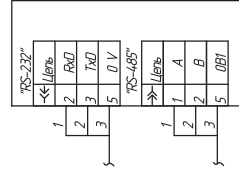
Адаптер интерфейса
