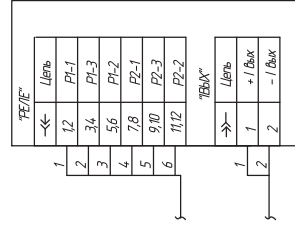
Устройство РТВ
