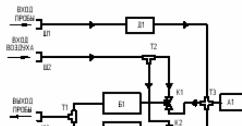
ж) газоанализаторы АНКАТ-4-10-06, АНКАТ-4-10-07,
