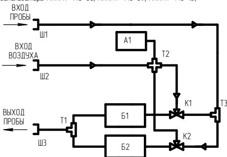
б) газоанализаторы АНКAT-4-10-08, АНКAT-4-10-09, АНКAT-4-10-10,
