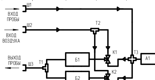
г) газоанализаторы АНКAT-4-10-03, АНКAT-4-10-04, АНКAT-4-10-05,
