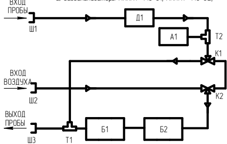
а) газоанализаторы АНКAT-4-10-01, АНКAT-4-10-02,
