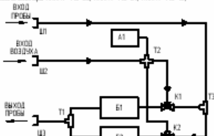
з) газоанализаторы АНКАТ-4-10-08, АНКАТ-4-10-09, АНКАТ-4-10-10,
